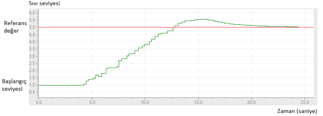
Şekil 1: Optimum katsayılarda sistemin cevabı
